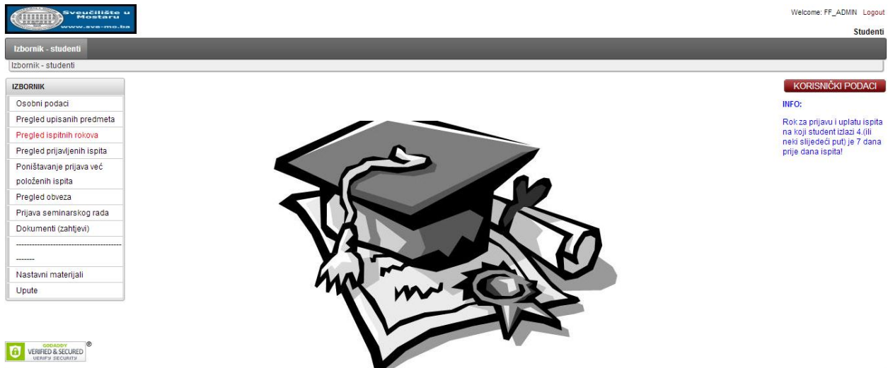
Slika 2 Početna stranica
