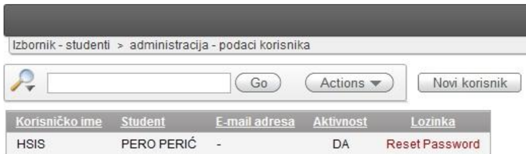
Slika 15 Korisnički podaci
